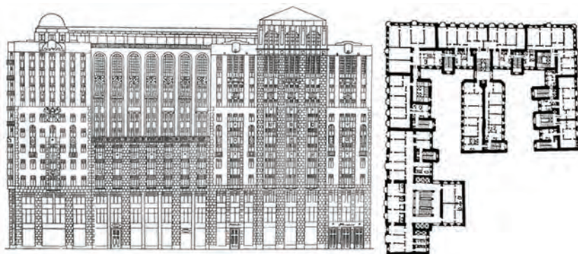
Рис. 6. Проект многофункционального «тучереза» фон Мекк на Тверской улице, 1912 года. Архитектор Машков. Из семейного архива
