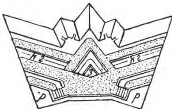
Илл. 5.1. «Бастионный фронт» французского инженера Пагана
