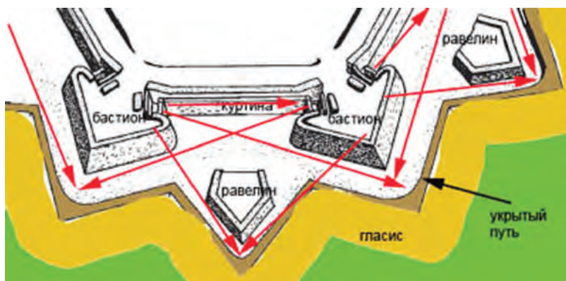
Илл. 9. Бастион Антуана де Вилля (1596–1656)
