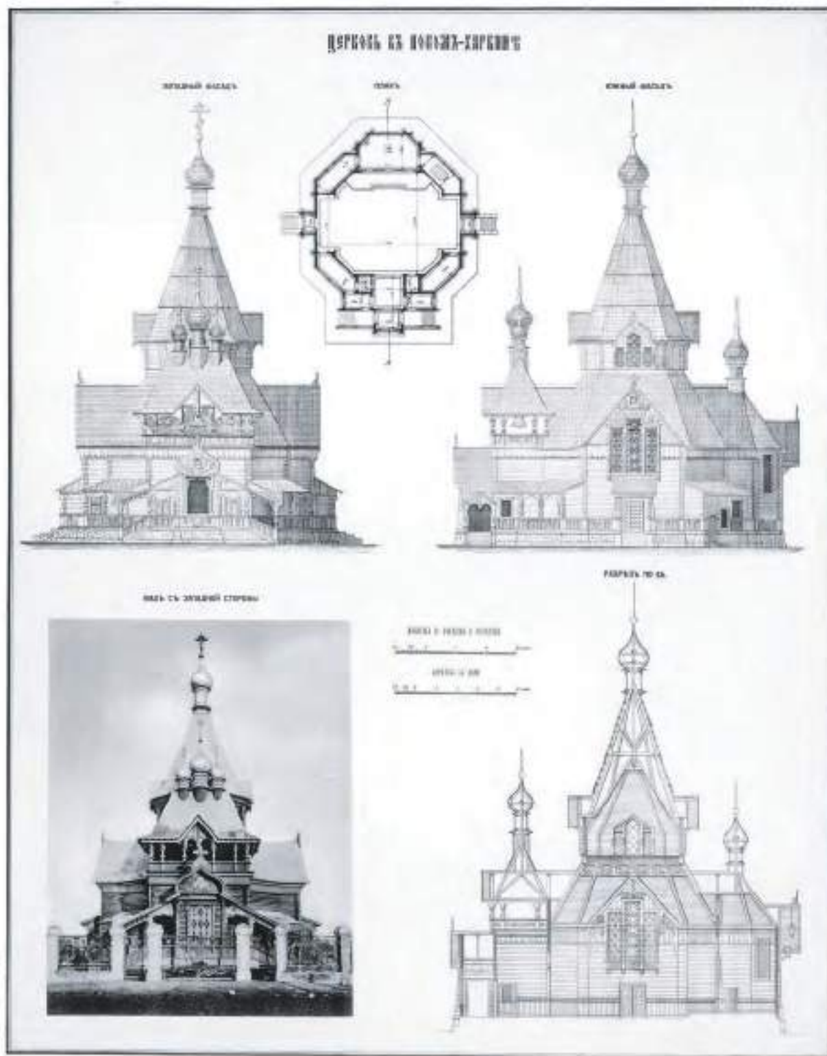
Проект Свято-Никольского собора архитектора И. В. Падлевского. Из Альбома сооружений и типовых чертежей Общества Китайской Восточной железной дороги 1903 г.
