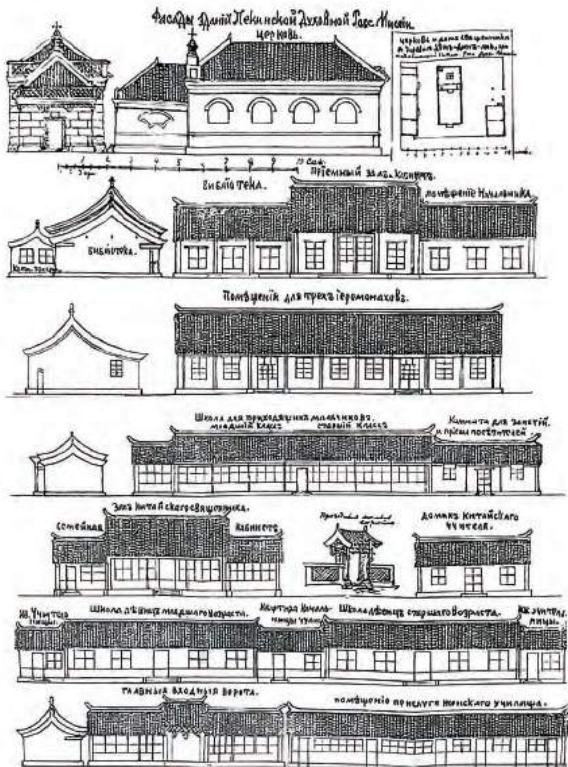
Чертежи зданий Русской духовной миссии в Пекине, выполненные иеромонахом Алексием (Виноградовым) в 1880-х гг.
