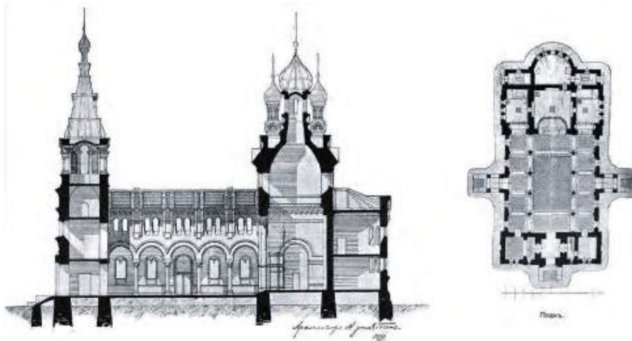
Проект Храма святителя Николая Мирликийского в Порт-Артуре
