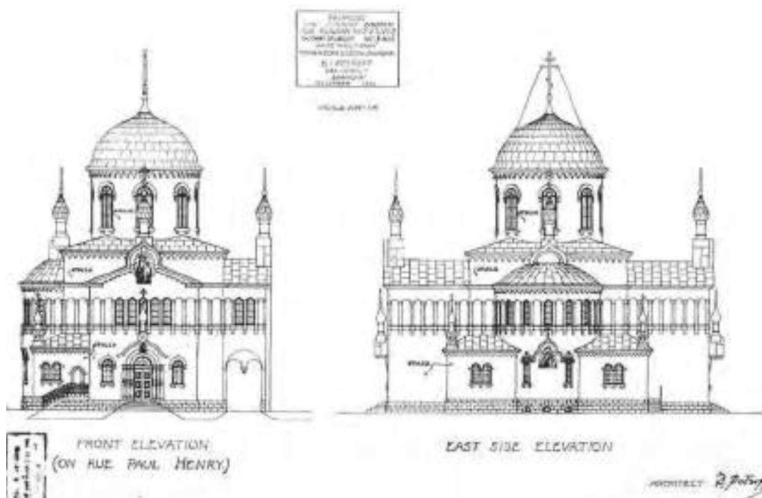
Проект собора архитектора Б. И. Петрова
