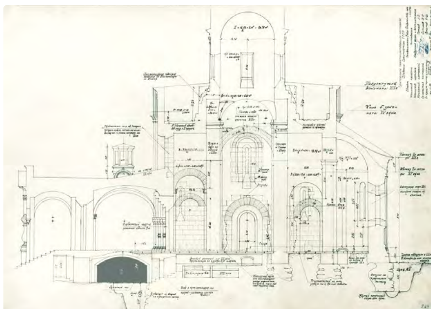
Рис. 22. Белокаменный Собор Андроникова монастыря, г. Москва. Продольный разрез и восст. интерьера. Центральная проектно-реставрационная мастерская Академии Архитектуры СССР. 1954 год. На чертеже отмечен проход из помещения под западной галереей в подполье, где находились захоронения. Представлена схема захоронений. Надпись: «Вход в месторасположение захоронений-усыпальницы заложен кирпичом»
