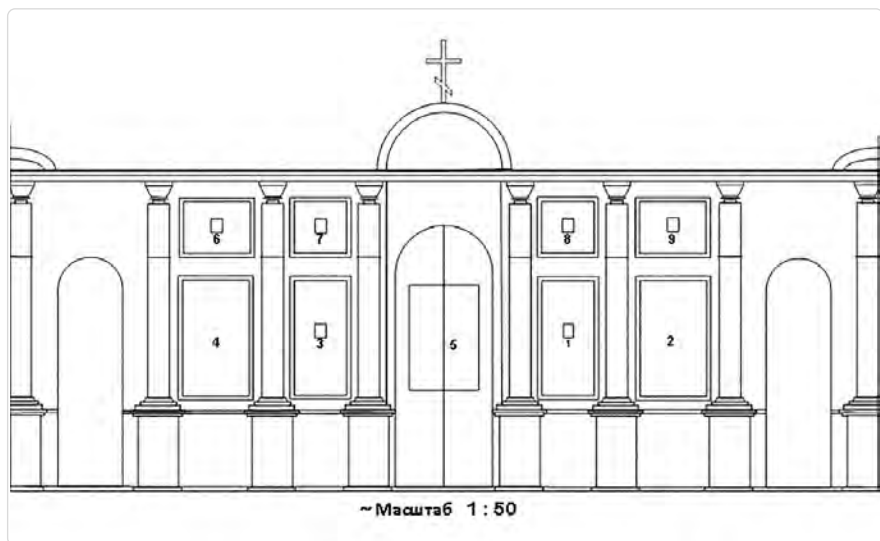
Рис. 16. Схема иконостаса Спасского собора. 1820 год.
