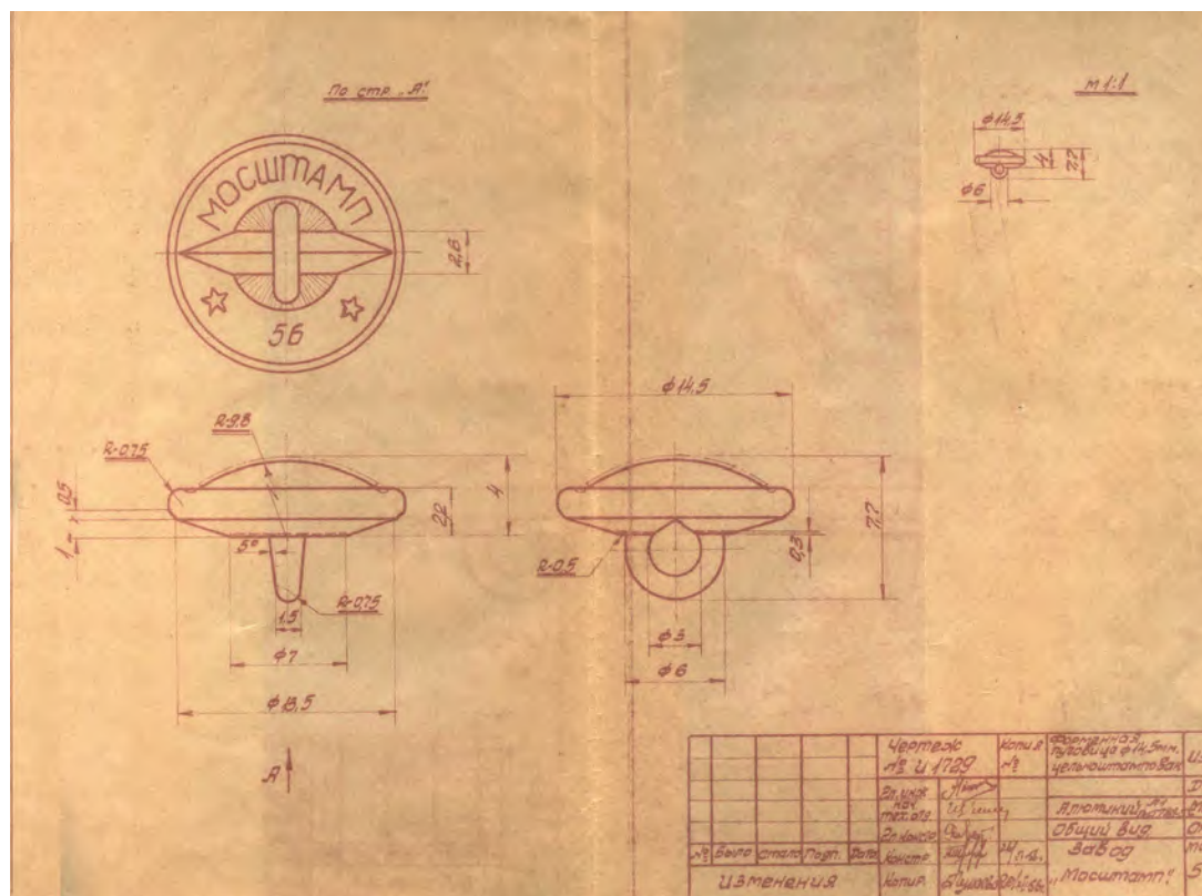
Проектный чертёж алюминиевой цельноштампованной пуговицы завода «Мосштамп». 1956 год
