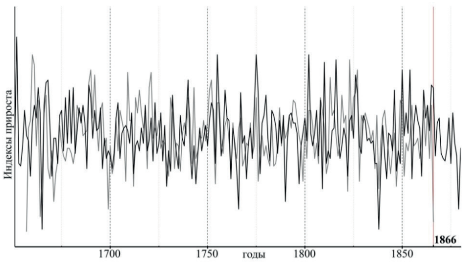
Рис. 3. Перекрестная календарная датировка ДКХ «КС» (серая линия) с ДКХ «IB_IC» (черная линия)
