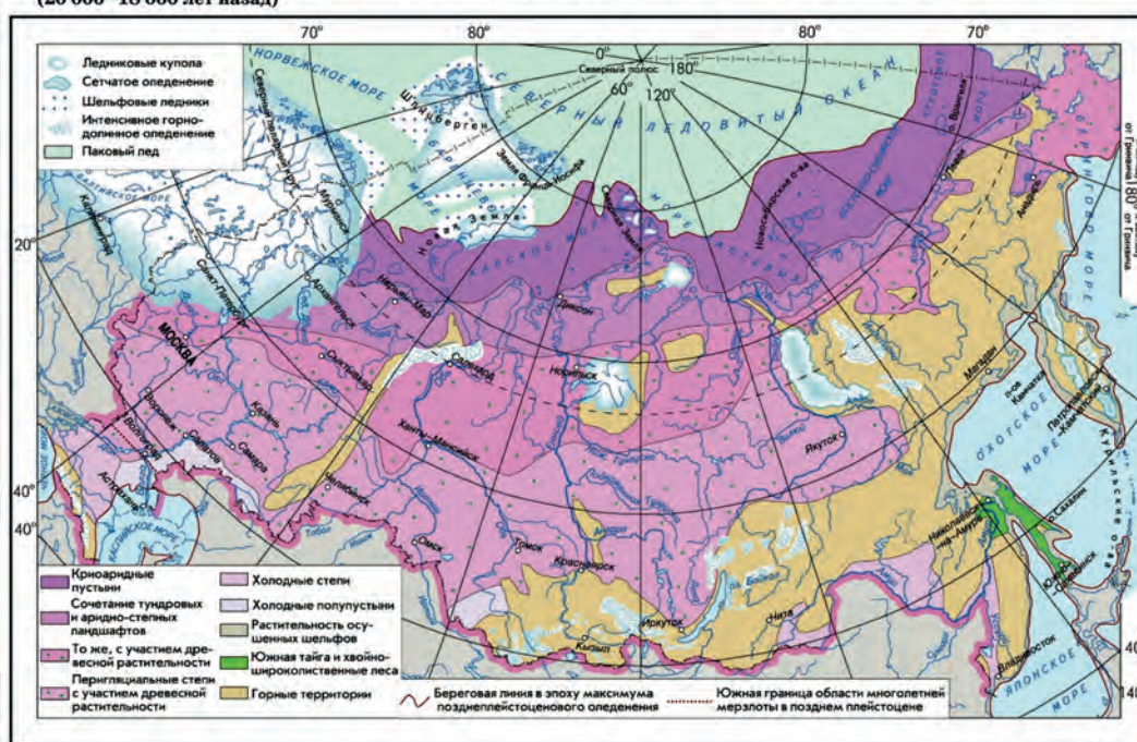
ФИЗИКО-ГЕОГРАФИЧЕСКИЕ ЗОНЫ В ЭПОХУ МАКСИМУМА ПОСЛЕДНЕГО ОЛЕДЕНЕНИЯ (20 000–18 000 лет назад)
