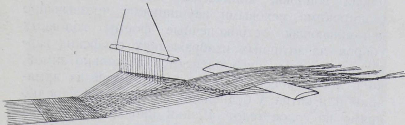
Схематический чертеж положения нитей при тканье. (Положение первое).
