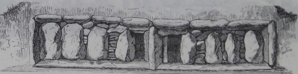
4) Prospect, 5) Grundtegning og 6) Gjennemsnit af en Jættestue med to Steenkamre ved Rödninge paa Møen.
