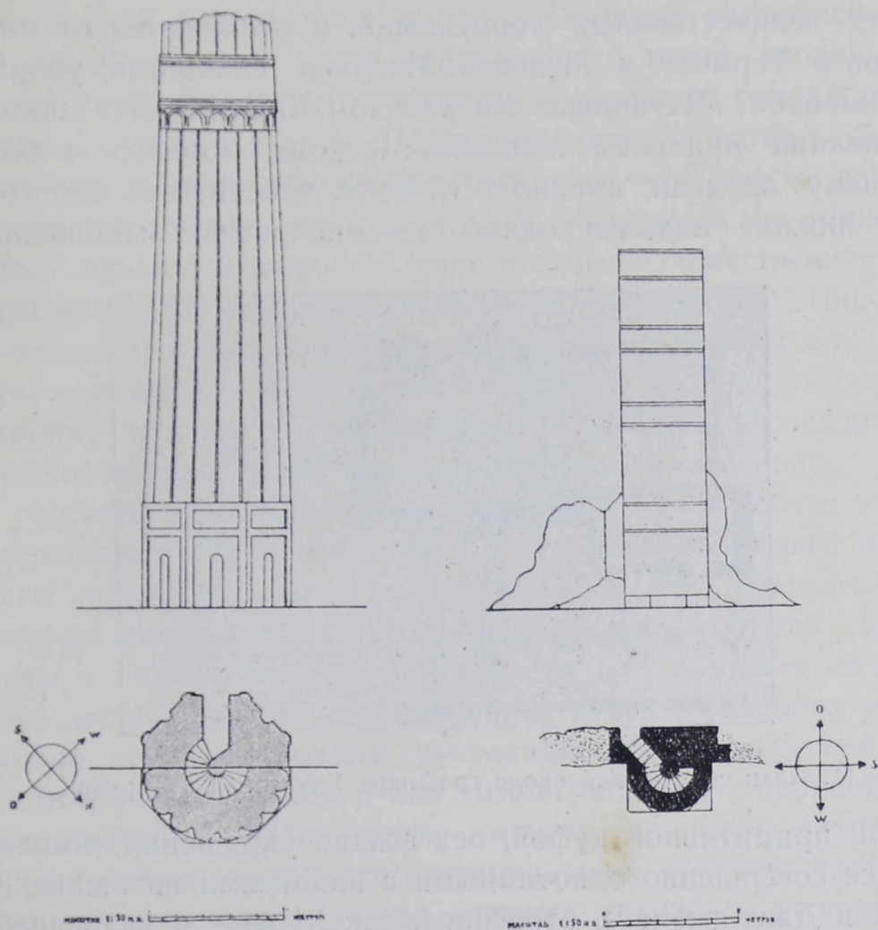
10. План термезского и жаркурганского минаретов.
