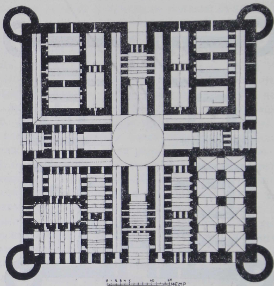
13. Кырк Кыз. План 2-го этажа.
