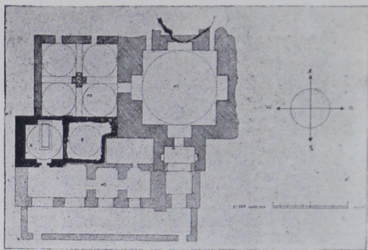
11. План сооружений около гробницы Хакими Аль Термези.
