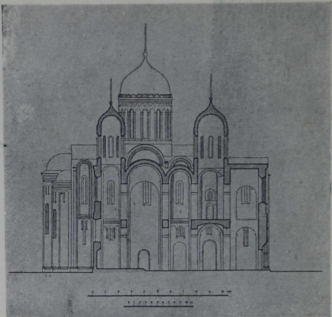
Рис. 10. Успенский собор. Разрез по северному нефу (обмер архитекторов Н. Н. Устинова и Г. К. Патрикеева).
