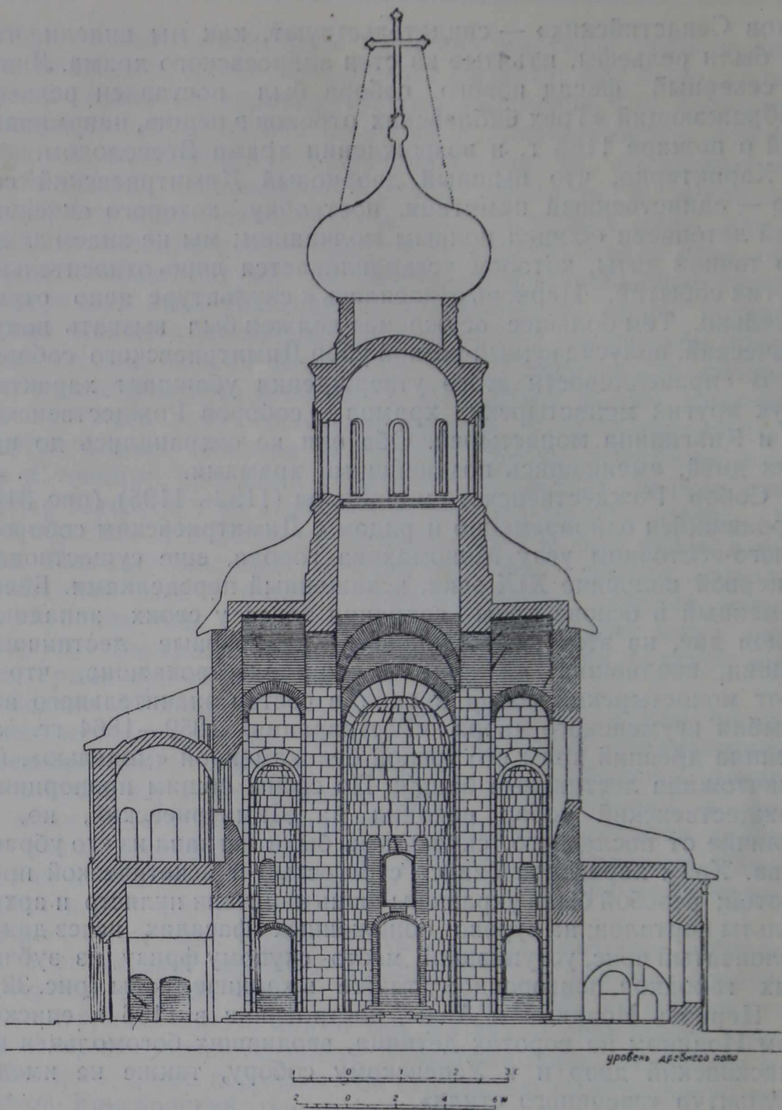
Рис. 31. Собор Рождественского монастыря. Разрез (чертеж Н. А. Артлебена).
