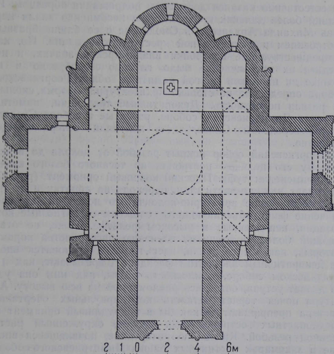
Рис. 43. Георгиевский собор в Юрьеве-Польском (1230—1234 гг.). План
