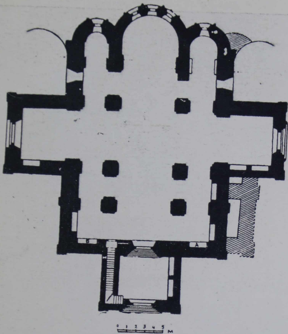
Рис. 35. Суздальский собор (1222—1225). План (по А. Д. Варганову).
