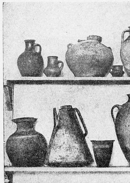
Рис. 4. Булгарская посуда — из глины В верхнем ряду правый крайний и в нижнем ряду левый крайний — глиняные.
