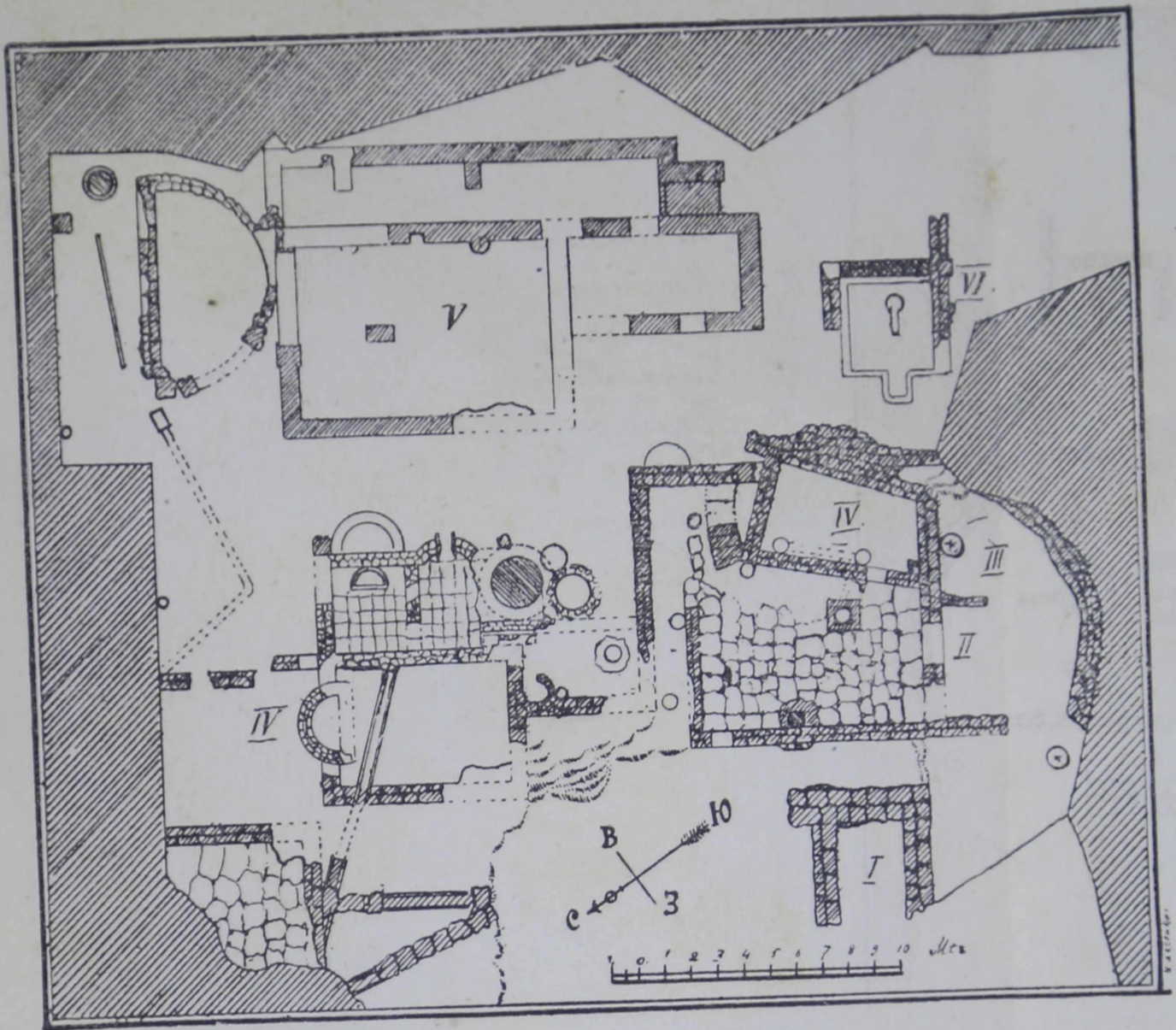
Рис. 8. План раскопки городища Пантикапея на горе Митридата 1
