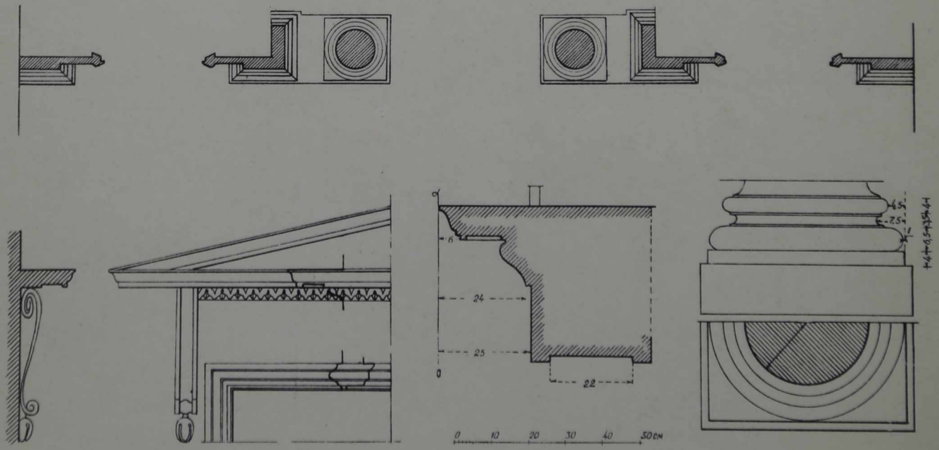
Парадная спальня. Перегородка. Обмер и реконструкция
