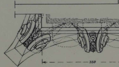
Парадная спальня. Капители колонны и пилястры. Обмер и реконструкция
